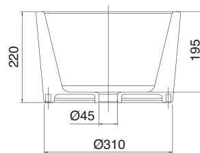
SEZIONE A-A
