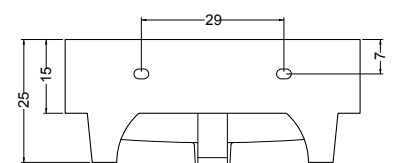
VISTA POSTERIORE
