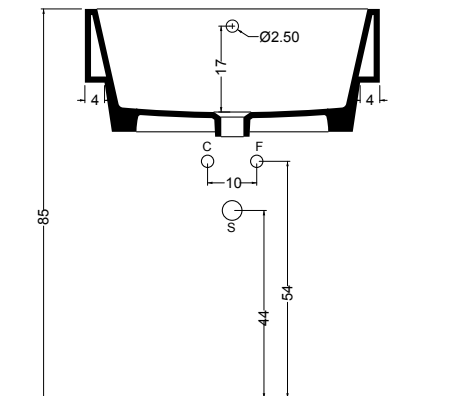
SEZIONE A-A
