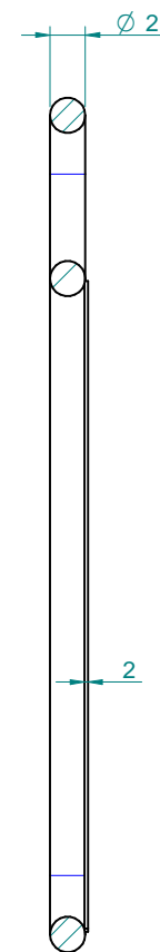
SEZIONE A-A
